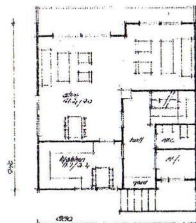
plan av 1ste. etasje.
